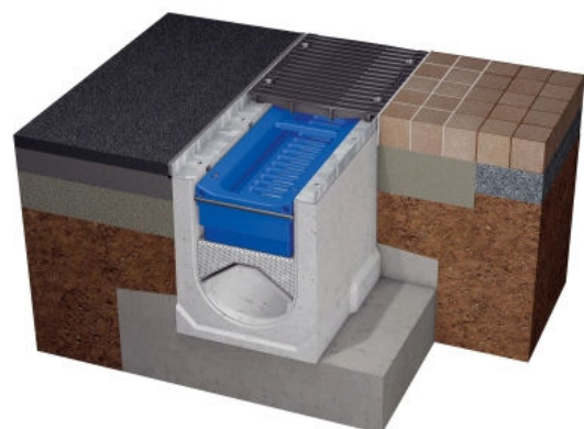
BIRCOpur® – Modularer Aufbau zur ökologischen Entwässerung
