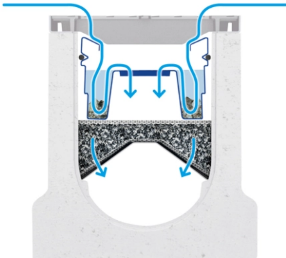
BIRCOpur® Systemschnitt, Aufbau
