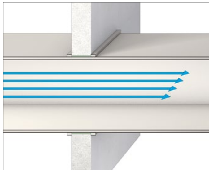
Wanddurchführung einer PROMATECT®-LS-Lüftungsleitung ohne Einbauteil
