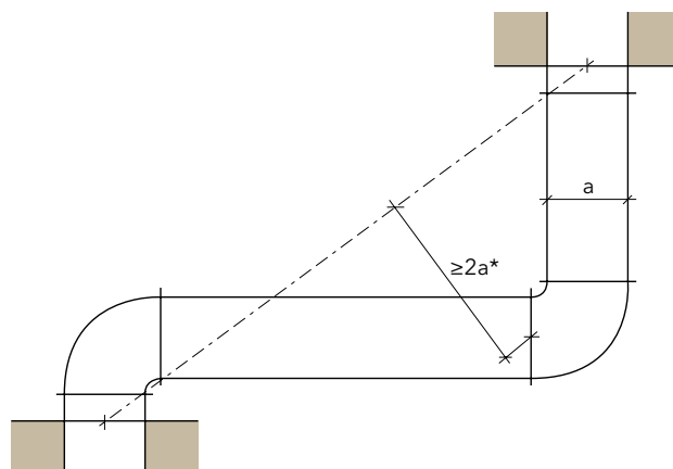
Bild 5.1: Begrenzung der Krafteinleitung mit Leitungsverzierung
