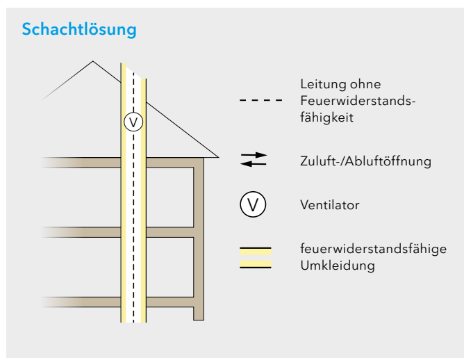
Abbildung 2: M-LüAR, schematische Darstellung, Abschnitt 2
