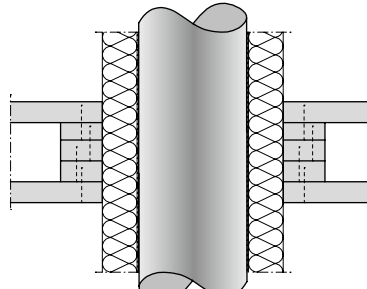
nichtbrennbare Rohre Rohrschott Beispiel Konstruktion 500.45
