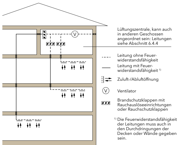
Bild 2.2: Schachtlösung
