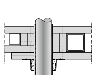
brennbare Rohre Rohrschott Beispiel Konstruktion 500.30
