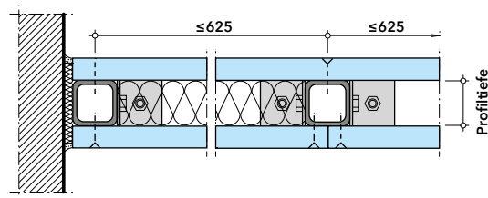
Horizontalschnitt mit Plattenstoß auf dem Stahlprofil
