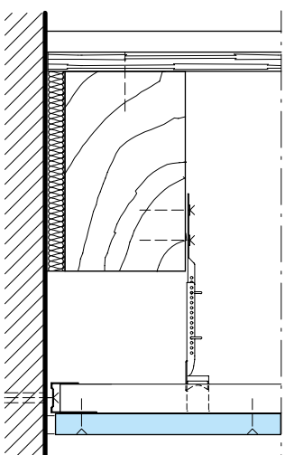
Querschnitt mit Wandanschluss
