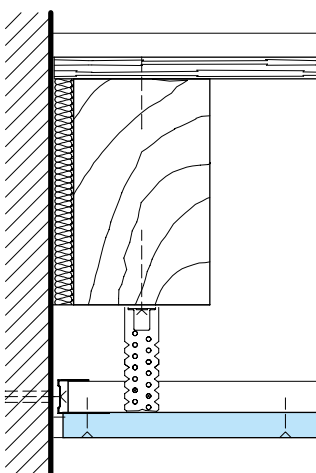
Querschnitt mit Wandanschluss
