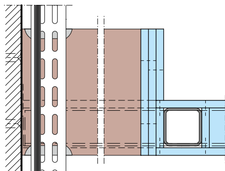
elektrische Installationen Kabelschott Beispiel Konstruktion 630.41
