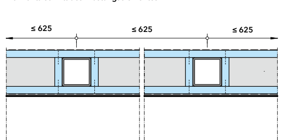
Horizontalschnitt des Brüstungselementes
