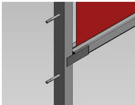
Fallstabführung BS-C-MQ1
