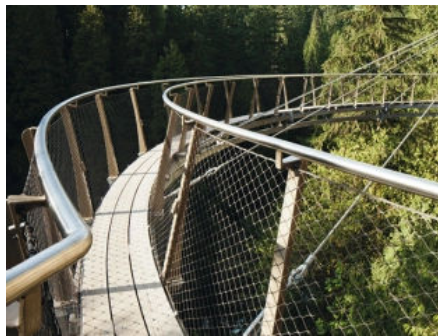
Klippenpfad Capilano Hängebrücke, Vancouver, Kanada
