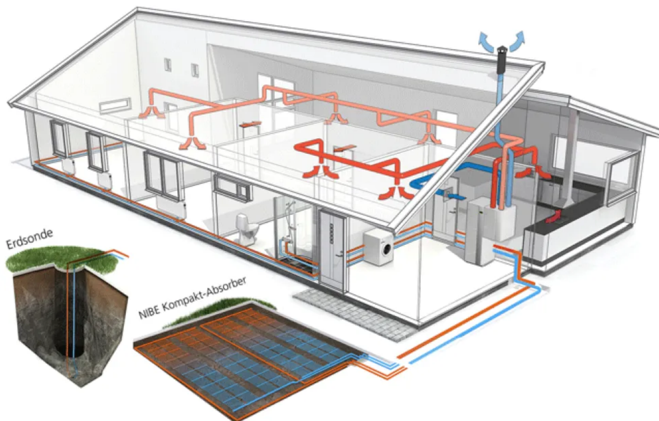
Systembeispiel in Verbindung mit einer NIBE Sole/Wasser-Wärmepumpe
