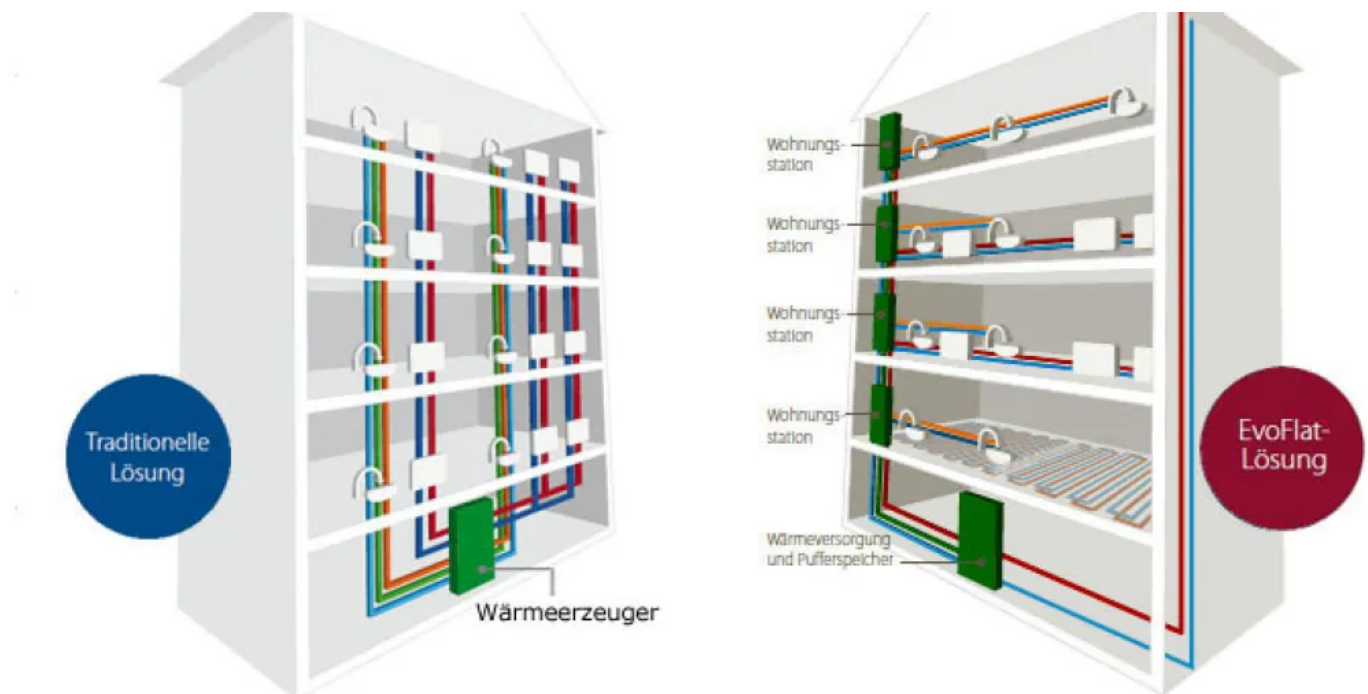
Traditionelle Anordnung eines Zentralheizungssystems mit zentraler Trinkwassererwärmung
