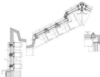
Schnitt Glashaussystem Variolux
