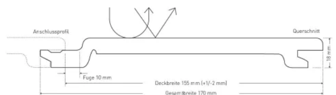
Fassadenprofil selekta REFINE
