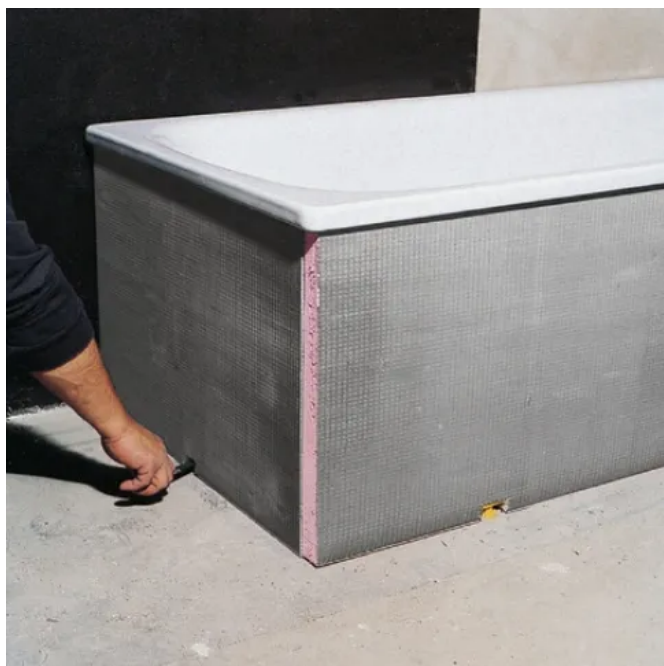
Austrotherm UNIPLATTE® Wannenelement
