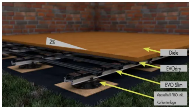
U2020 Profilsystem mit Verstellfüßen auf Korkunterlagen, Variante Slim
