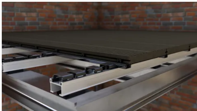
U2020 Profilsystem auf Stahlträger
