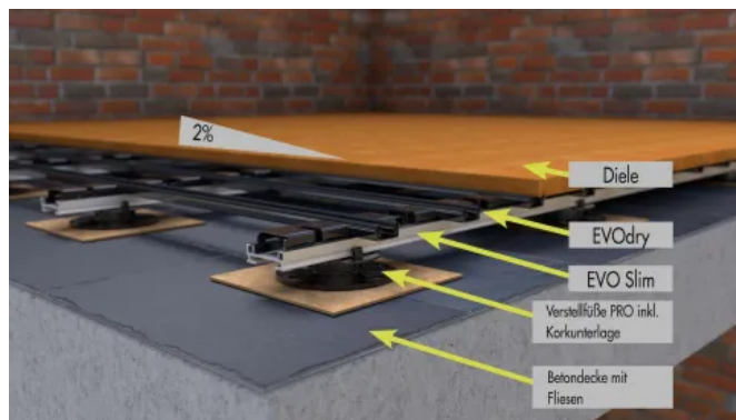
U2020 Profilsystem mit Verstellfüßen auf Betondecke
