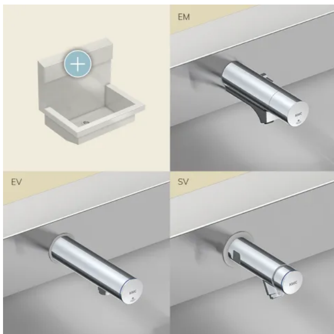
3 mögliche Armaturenvarianten: hydraulische oder elektronische Wandventilen sowie elektronische Wandbatterie mit Temperaturwahlhebel
