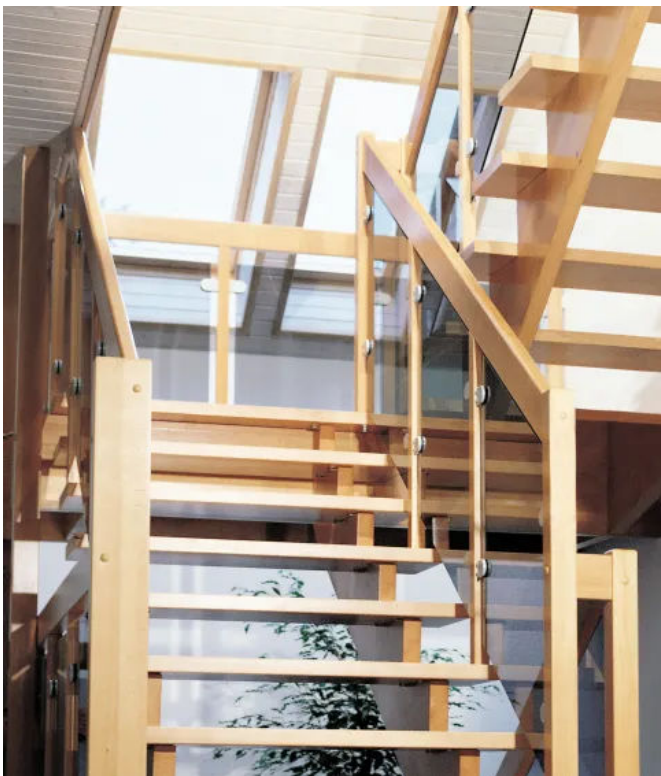
Casa CA 107, Wangen, Stufen und Podest: Buche massiv, Handlauf: Buche massiv, Geländerfüllung: ESG-Glas
