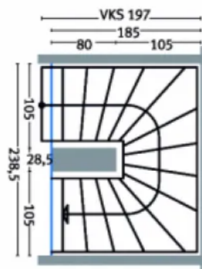
2/4 gewendelte Treppe
