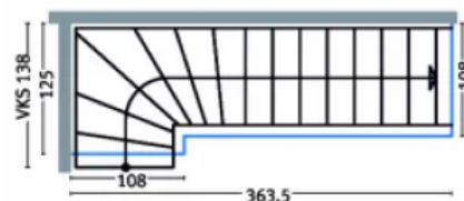
1/4 gewendelte Treppe
