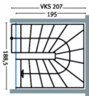
1/2 gewendelte Treppe
