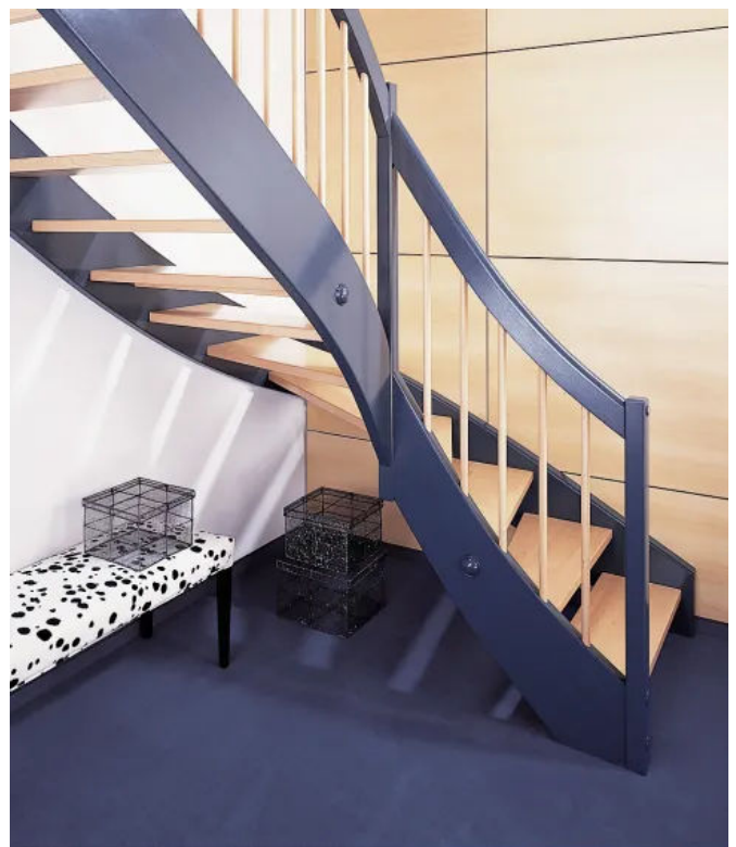
Meran ME 106, Wangen und Handlauf: Esche massiv, anthrazitgrau, Stufen: Buche massiv, Geländerstäbe: Buche massiv, Typ S
