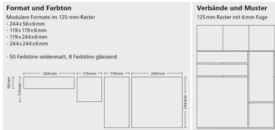
Gestaltungsparameter StoCera 100
