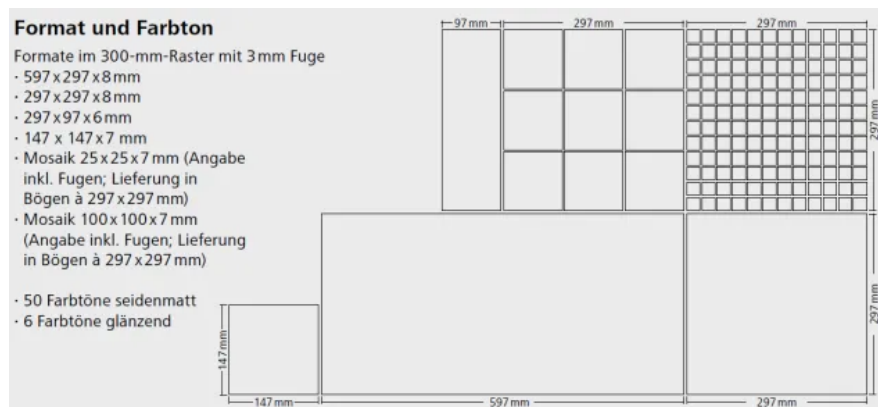
Gestaltungsparameter StoCera 200
