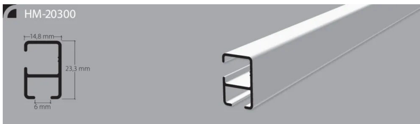
Profil HM-20300 I
