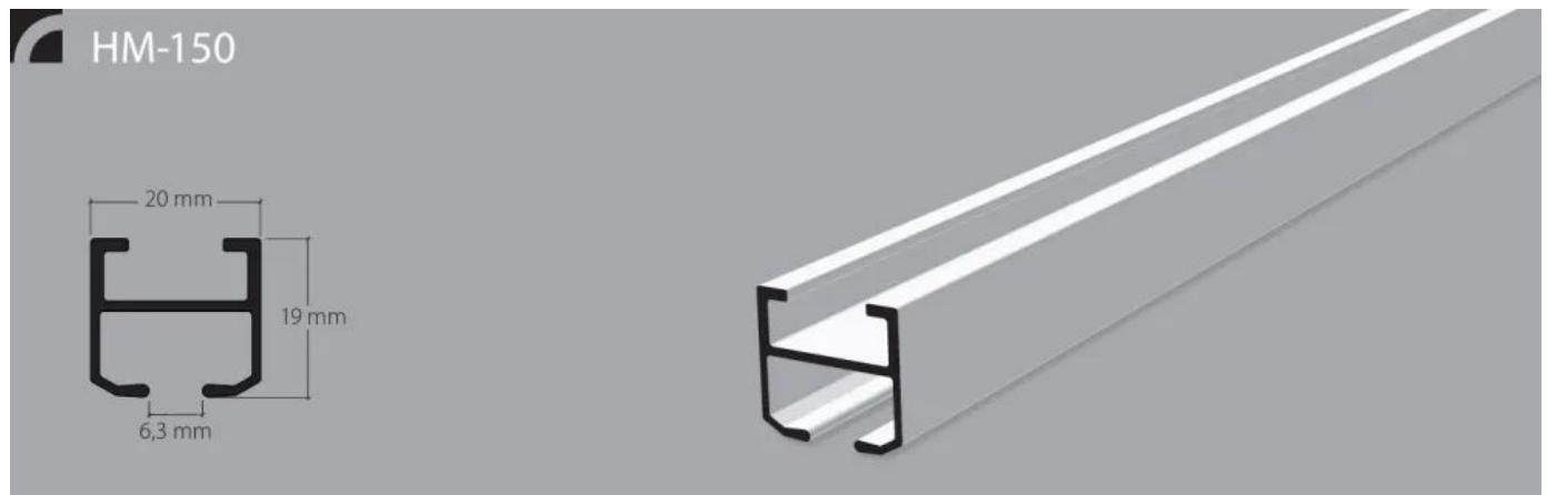
Profil HM-150 | Vorhangprofil für Decken und als Rauntrenn-System verwendbar
