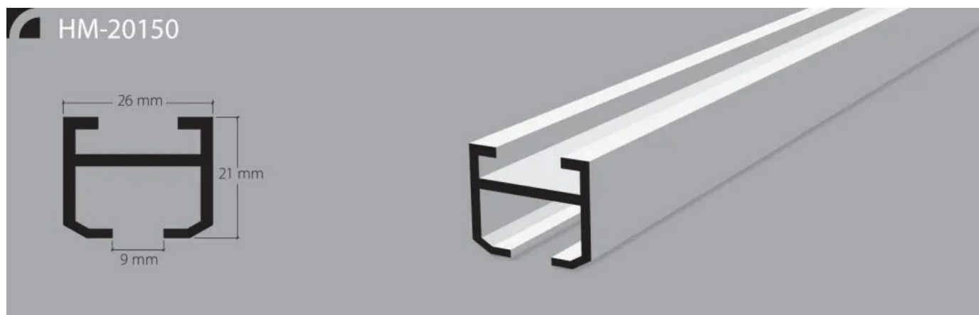
Profil HM-20150 | Balkon-Vorhangprofil
