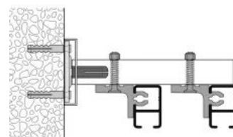
Profil HM-20300 I Wandträger 2-Lauf wird an die Decke geschraubt, Profile eingeklickt
