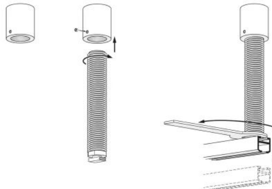
Profil HM-20150 | abgehängte Befestigung
