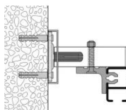
Profil HM-20300 I Wandträger 1-Lauf wird an die Decke geschraubt, Profil eingeklickt
