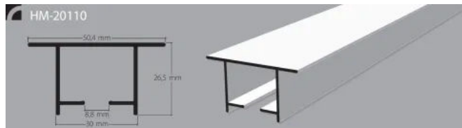
Vorhangprofil HM-20110 | für den Außenbereich mit Biegeradien ab 300 mm
