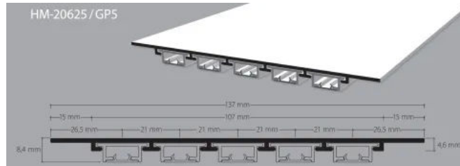
Profil HM-20625 | Flächenvorhangprofil-System, bis 5-läufig frei wählbar, komplett mit Profil, Gipschutzband eingelegt und haftgrundbehandelt zum Eingipsen
