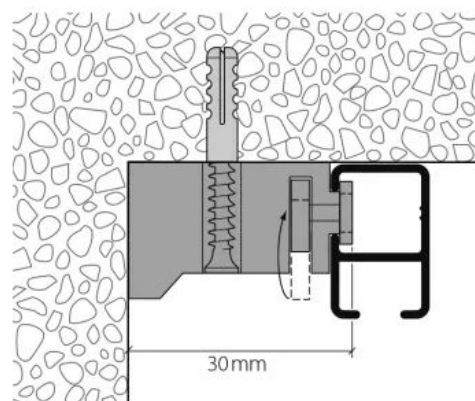
Profil HM-20300 I Deckenträger 30 mm wird an die Decke geschraubt, Profil eingeklickt
