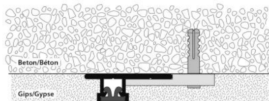
Unterputz-Profil HM-20190 | an Betondecke befestigt mit eingelegtem Gips-Schutzband während des Verputzens
