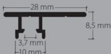
Profil HM-20190 | Bilder-Deckenprofil für die Unterputzmontage, haftgrundbehandelt, mit im Profil eingelegten Gips-Schutzband
