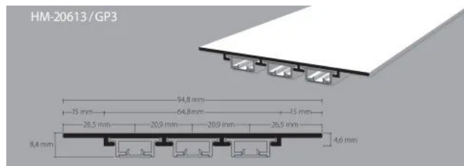
Profil HM-20613 | Flächenvorhangprofil-System, bis 3-läufig frei wählbar, komplett mit Profil, Gipschutzband eingelegt und haftgrundbehandelt zum Eingipsen
