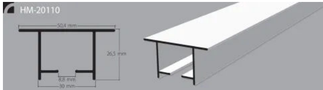
Vorhangprofil HM-20110 | für den Außenbereich mit Biegeradien ab 300 mm
