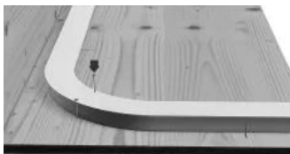
... Profil auf Montagebänder geklippt, mit Nägeln fixiert ...
