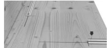
... Schal Brett wird vermaßt, vorgelochte Montagebänder befestigt ...
