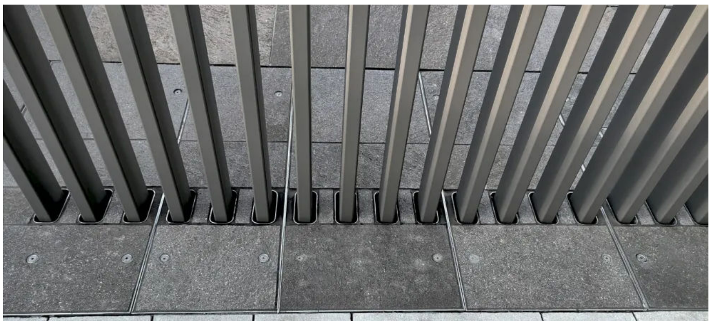
FancyFence Zaun | die Pfosten gleiten in einen im Boden integrierten Stahlbetonschacht
