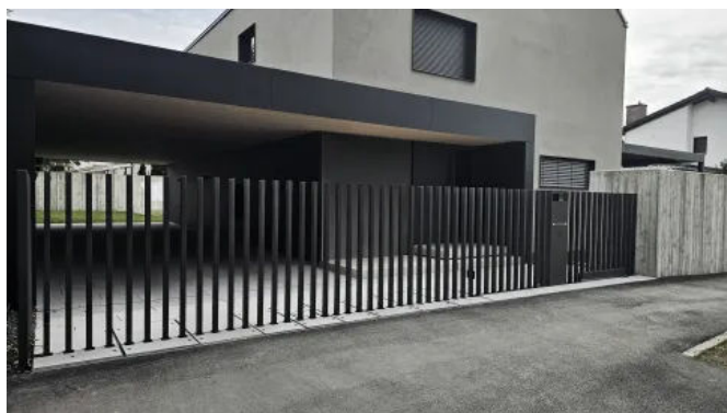
Private Zaun- und Toranlage | mit versenkbaren Torpfosten und schwenkbarem Gartentor
