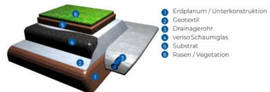
Systemskizze Drainageschicht für Sportplätze
