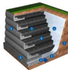
Systemskizze Hangsicherung
