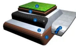
Systemskizze Drainageschicht für Sportplätze
