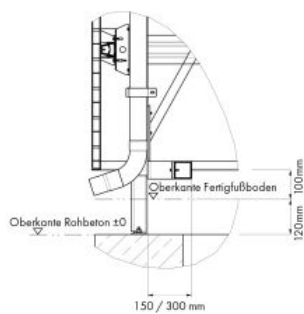
Optionaler Rammschutz
