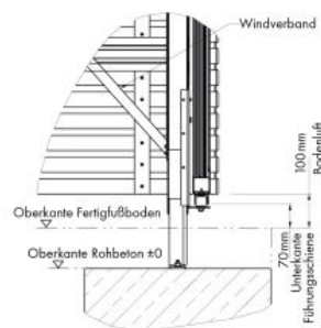
Auslaufende Schiebetür
