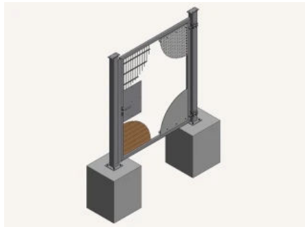
Flügeltor einflügelig
