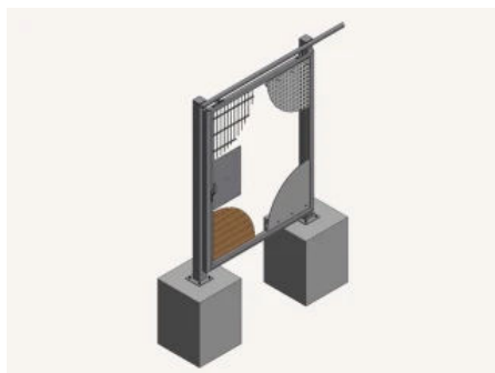
Hängeschiebetor einflügelig
