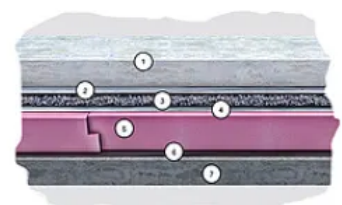
Austrotherm Parkdach Aufbau
