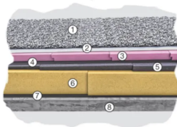
Austrotherm Duodach Aufbau
