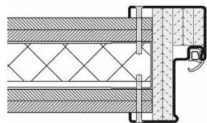
Senkschraubenbefestigung (Leichtbauständerwand)
