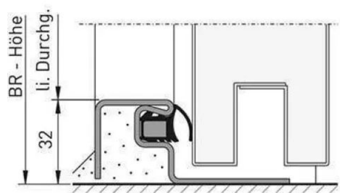
Anschlagdichtung
