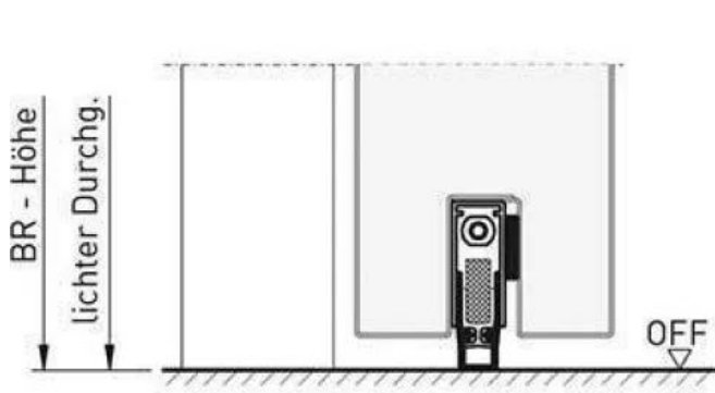
Absenkbare Bodendichtung
