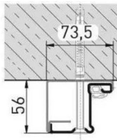
Typ 5.1 Dübelmontage vor der Öffnung (Mauerwerk/Beton)
