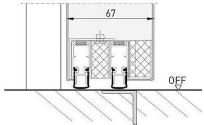
Doppelte absenkbare Bodendichtung (für hochschalldämmende Türen)
