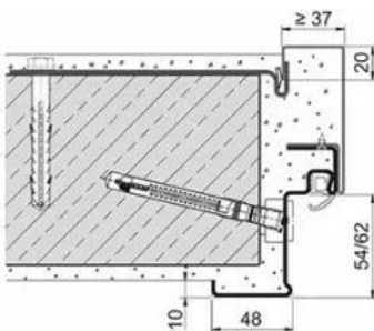
Eck-/Gegenzarge für 62er Türen Dübelmontage mit Aufschiebeanker (Mauerwerk/Beton)
