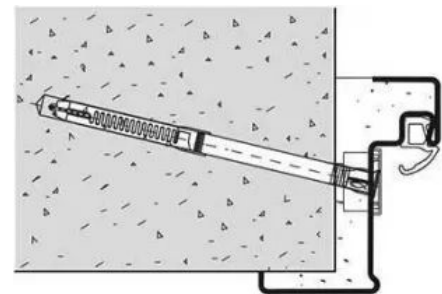
Dübelmontage (Porenbeton)
