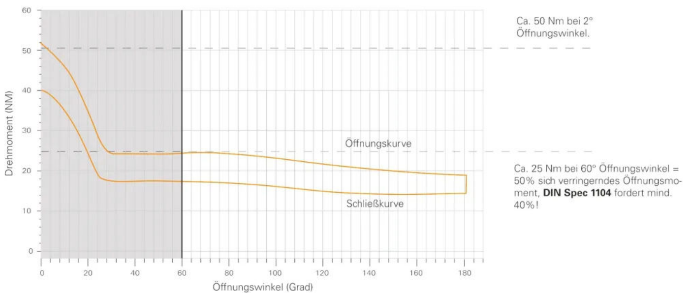
Drehmomentverlauf beim GTS 640
