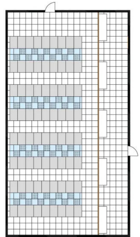
■ = Servertrennwände ■ = Server ■ = Kaltgang Abtrennung eines Wartungsganges mit DataSafe
