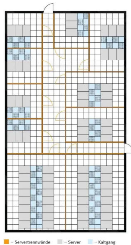
Unterteilung einzelner Serverbereiche mit DataFlex
