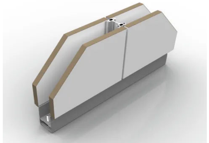
T10 Vollwand-System
