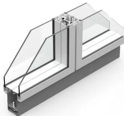
T34 Glas-Systemtrennwand
