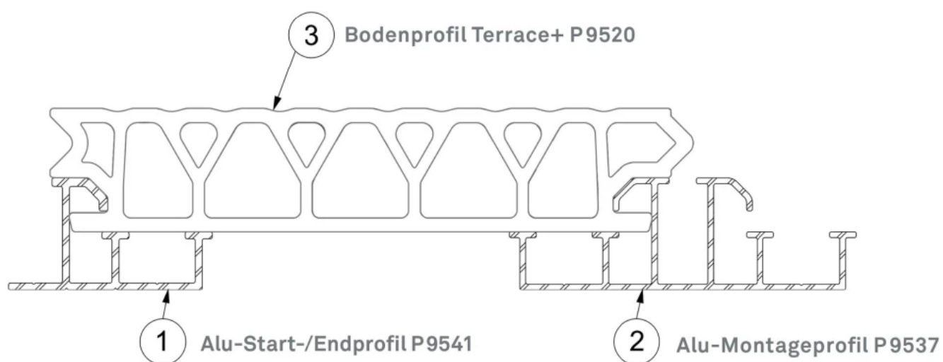
Profilschnitt Terrace+
