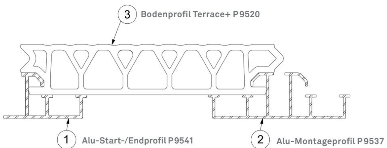
Profilschnitt Terrace+
