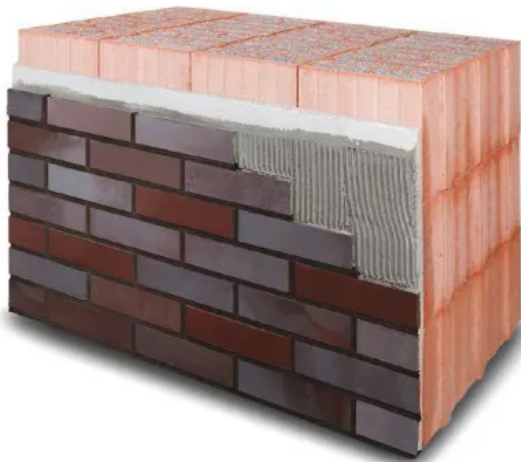
Einschalige Wandkonstruktion aus verfüllten Poroton-Ziegeln und Terca Riemchen ohne zusätzliche Dämmung.
