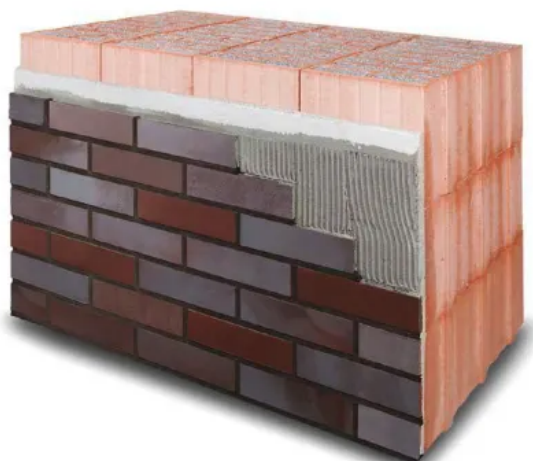
Einschalige Wandkonstruktion aus verfüllten Poroton-Ziegeln und Terca Riemchen ohne zusätzliche Dämmung.
