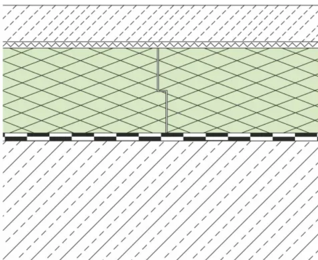
Ausführung Parkdach
