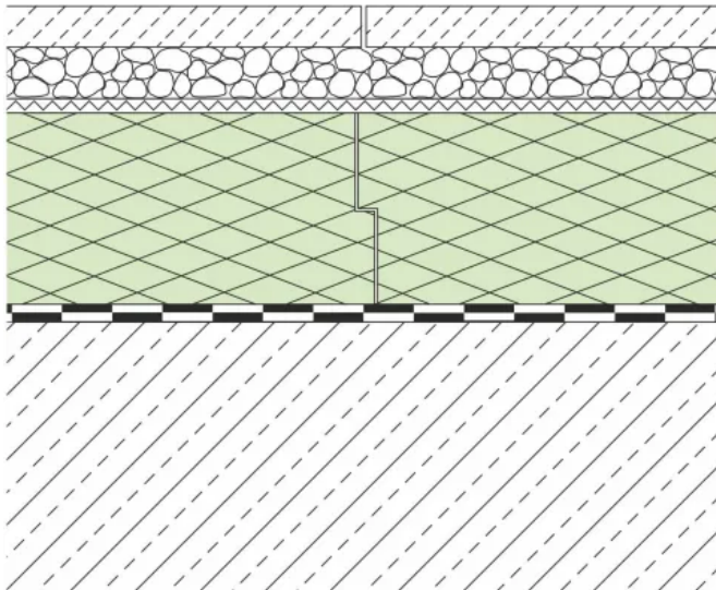
Konstruktionsbeispiel Terrassendach
