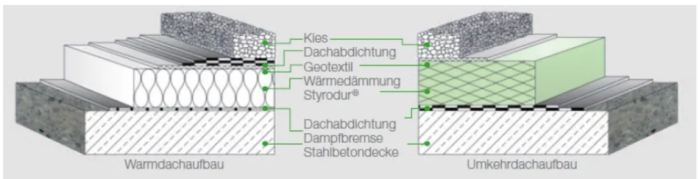
Vergleich von Warmdach- und Umkehrdachaufbau
