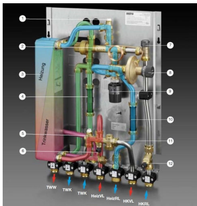
Trinkwasserbetrieb Regudis W für Heizkörperanbindung
