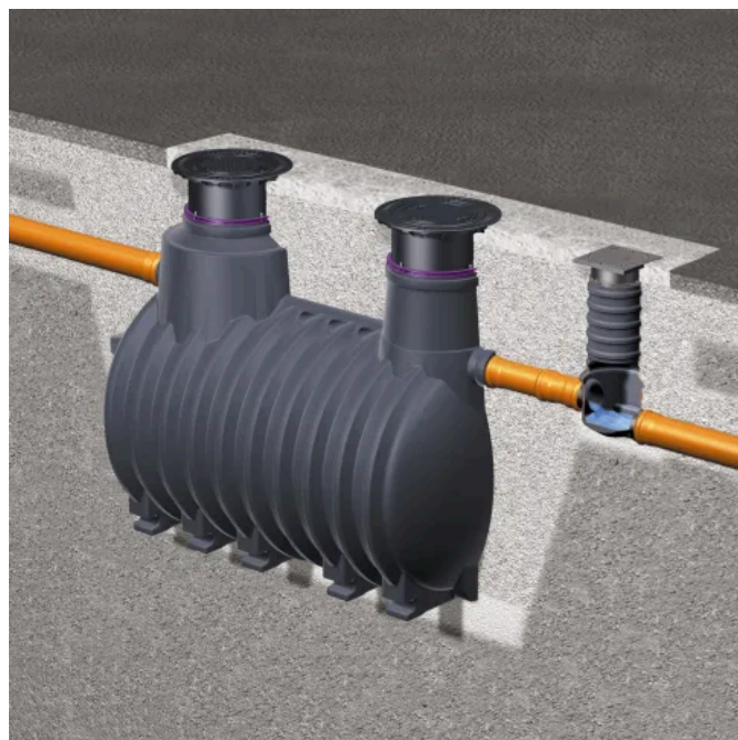
Stärkeabscheider EasyStarch ground NG 2 für den Erdeinbau
