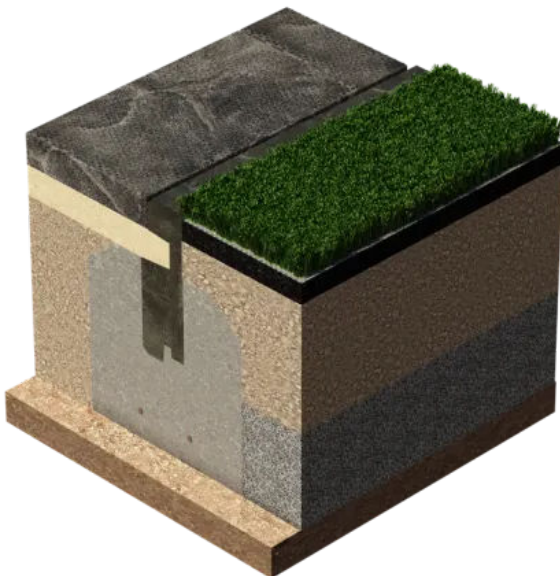
Anwendung als Kantenstein
