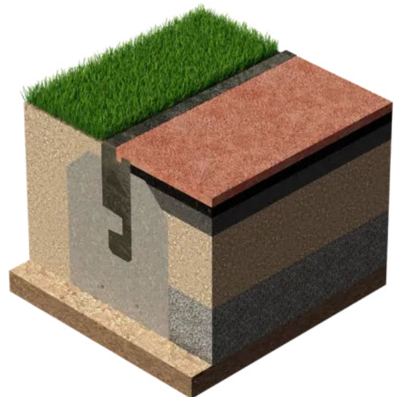
Anwendung als Einfassungsbord
