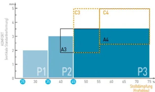
P1, P2, P3 : Kraftabbau-Klassen für punktelastische Böden gemäß EN 14904
