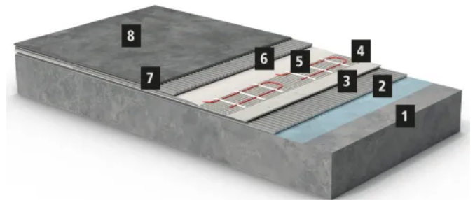
Verlegung elektrischer Heizsysteme mit Sopro Fließspachtelmassen
