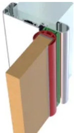
Fingerklemmschutzelement Touchguard plus – Typ 715
