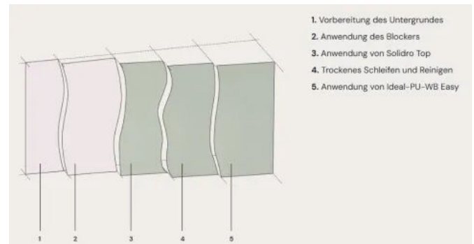
Solidro - Systemaufbau 3, für einfache Wände
