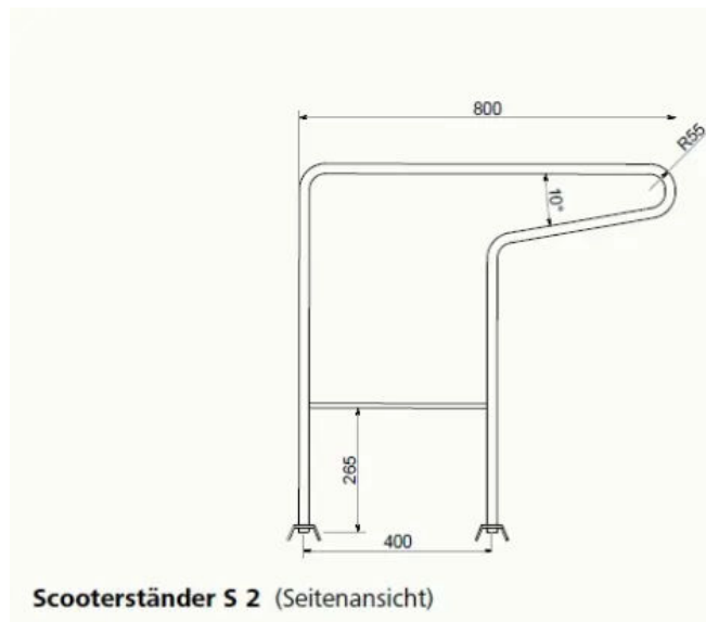
Maße ilco Scooterparker Modell S 2
