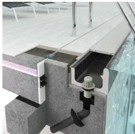
System Wiesbaden, hochliegend
