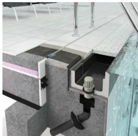
System Wiesbaden Stil, hochliegend
