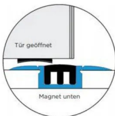
Funktionsprinzip der Alumat Magnet-Türschwellen
