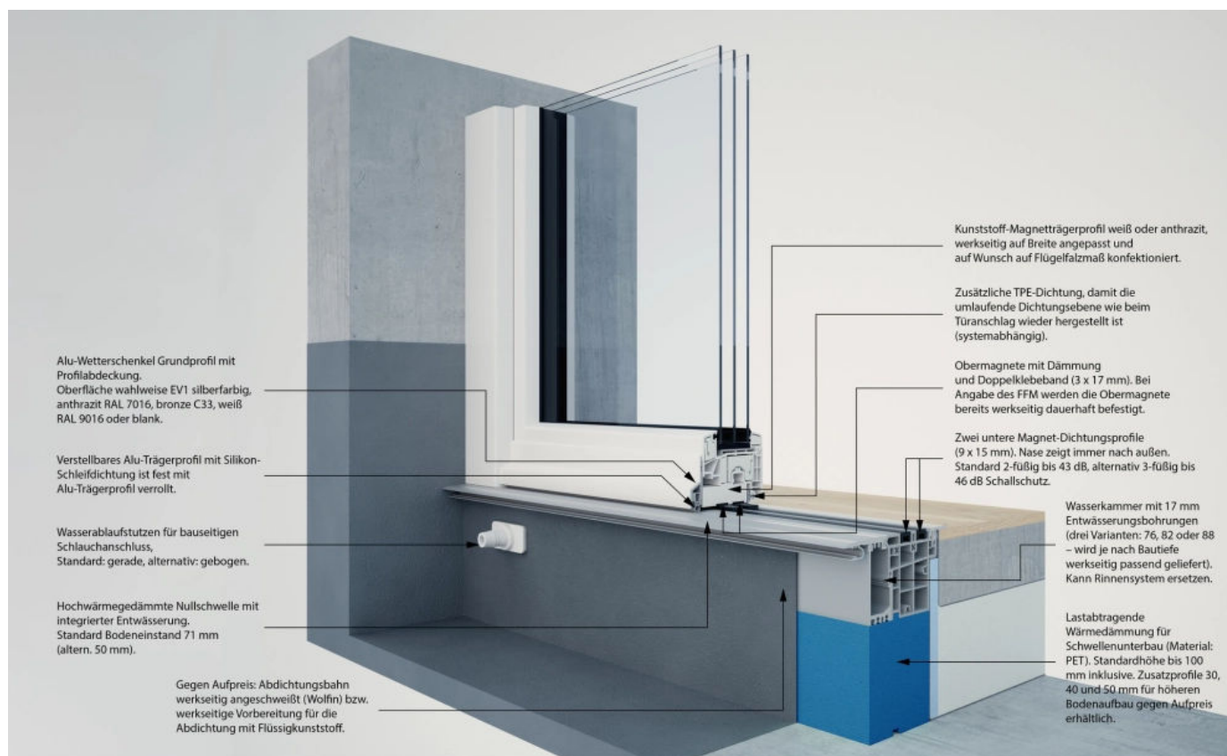
ALUMAT-Nullschwelle
