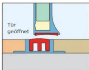
Magnet ist unten, der Durchgang bleibt absolut barrierefrei
