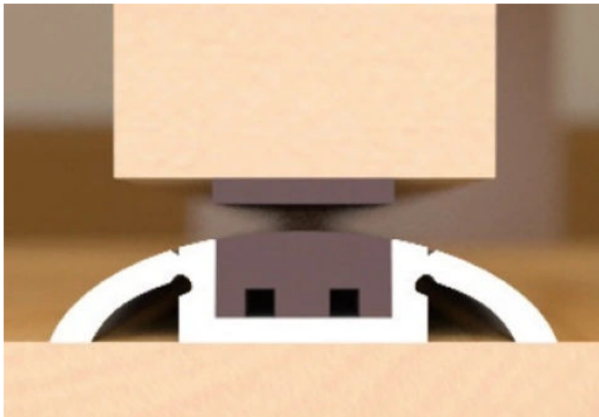
Standard-Aluminium-Bodenprofile
