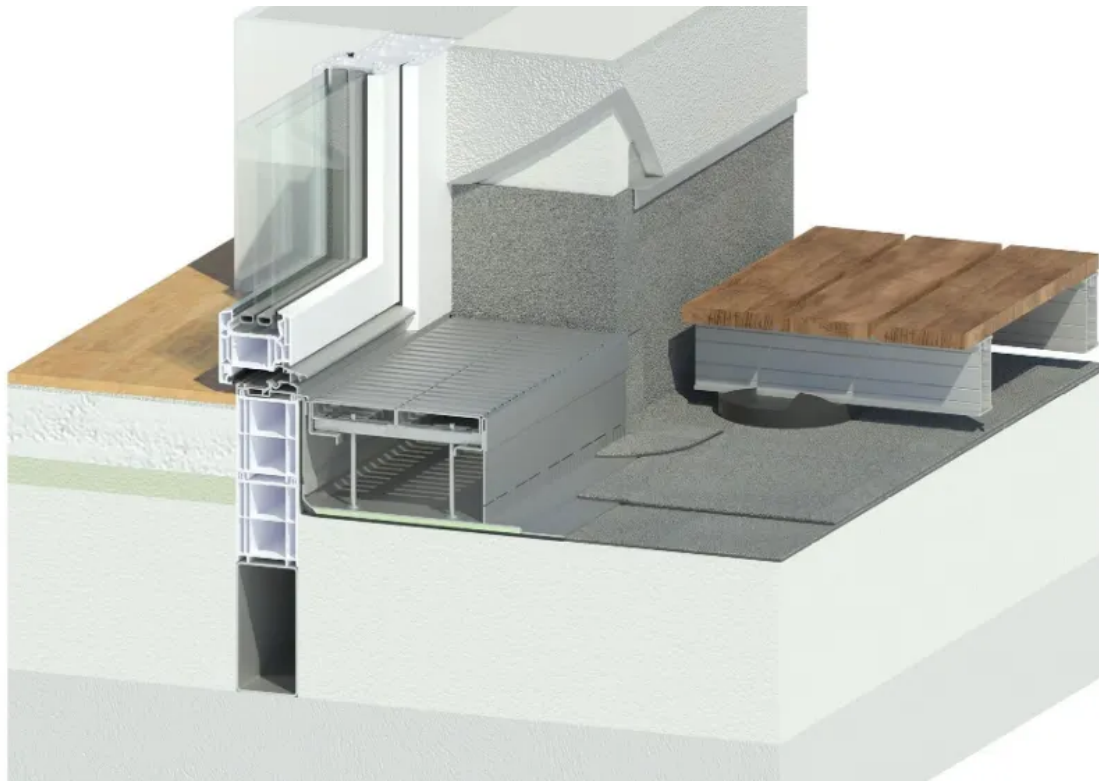
Barrierefreie Fassadenrinne INNORIN® F für den wärmebrückenfreien Anschluss an begehbaren Flachdächern
