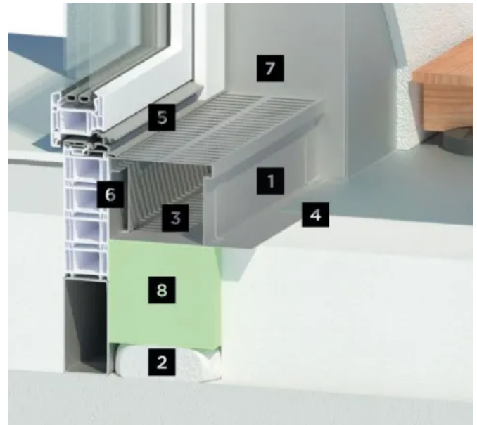
Barrierefreie Fassadenrinne INNORIN® F für den wärmebrückenfreien Anschluss an begehbare Flachdächern
