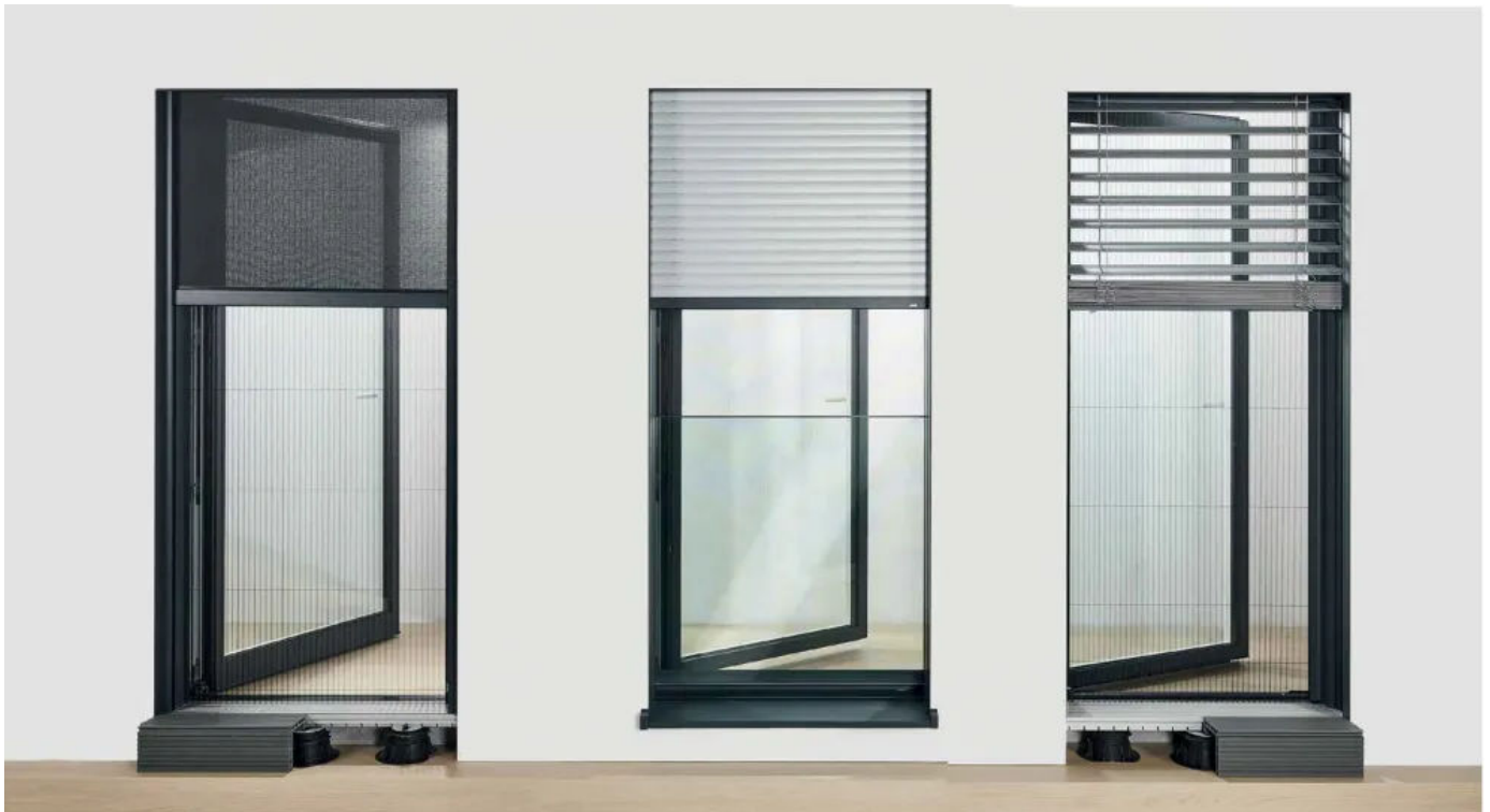
Sonnenschutz Varianten Zip-Design Screen | Rollläden | Raffstore
