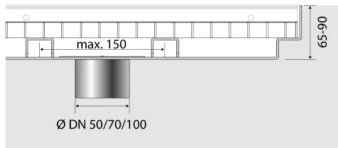
Querschnitt: Schmutzfangwanne Typ 5022+
