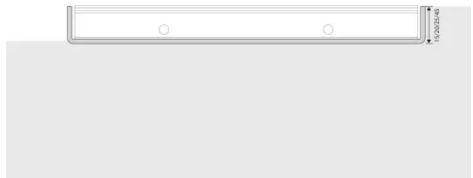
Querschnitt: Schmutzfangwanne Typ 5512, 5517, 5522, 5542
