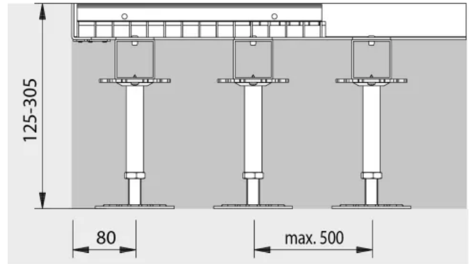
Spezialrahmen mit Unterkonstruktion Ausführung A
