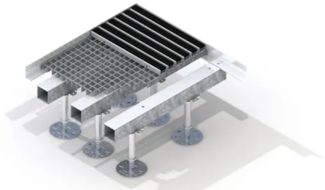
Unterkonstruktion Ausführung A
