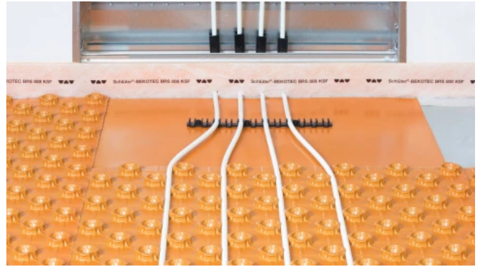
Die Ausgleichplatte Schlüter-BEKOTEC ENFGK-PS wird vor Heizkreisverteiltern eingesetzt, um die Montage der Heizrohre im Verteilerschrank zu erleichtern. Die Platte ist rückseitig selbstklebend und mit Schutzfolie versehen.
