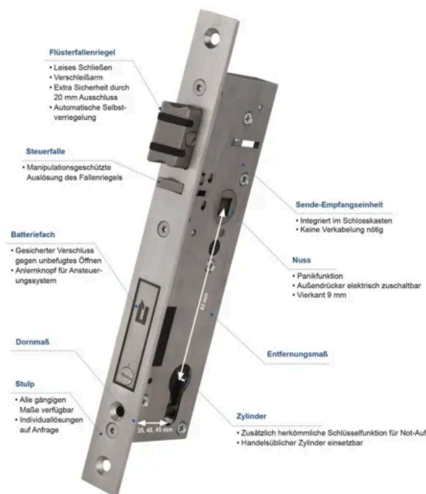
ÜLock-B: Funk-Sicherheitsschloss mit automatischer Selbstverriegelung
