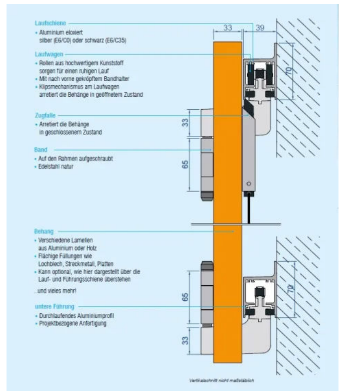
Schiebefaltladen Standard 30 – Vertikalschnitt
