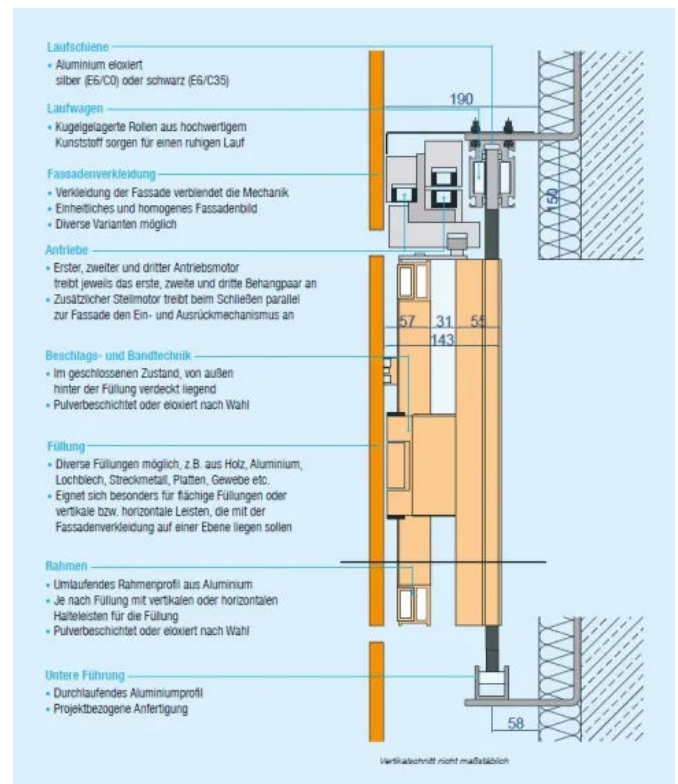
Schiebefaltladen Premium 70 – Vertikalschnitt
