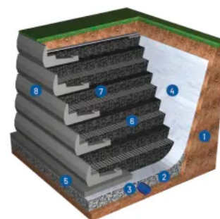
Systemskizze Hangsicherung
