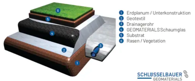
Systemskizze Drainageschicht für Sportplätze
