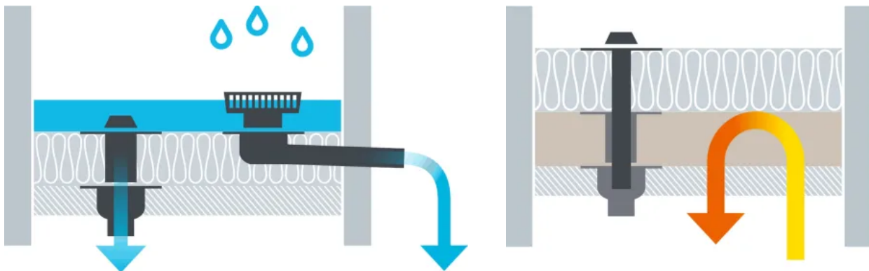
Nachrüsten der zusätzlichen Notentwässerung für eine normgerechte Entwässerung
