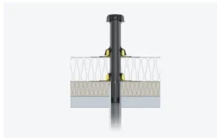
E. Für Be- und Entlüftung in das bestehende Rohr: SitaVent Sanierungslüfter
