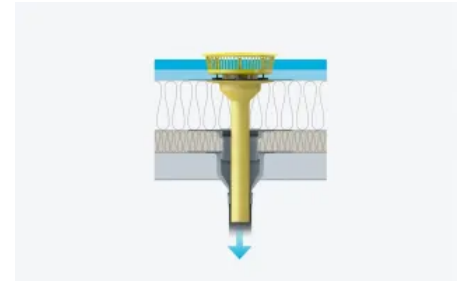
C. Für die Entwässerung in das bestehende Notentwässerungssystem: SitaSani
