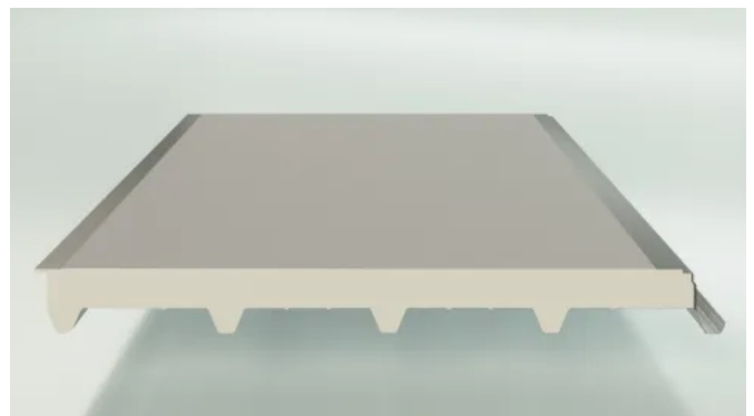
Isodeck PVSteel PU (Polyurethan)
