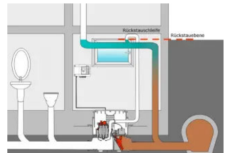
Notfall: Rückstau
