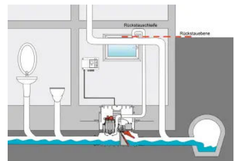
Normalbetrieb: Keller-Entwässerung
