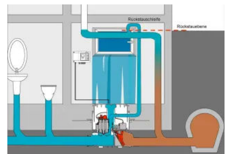
Extremfall: Kellerüberflutung
